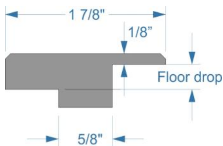
LTMU T-mould, uneven
