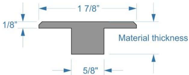
LTML T-mould, large
